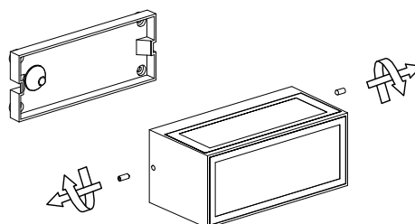
2. Untie side screws
