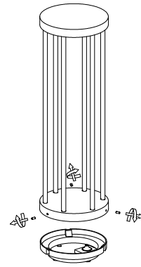
2. Untie side screws
