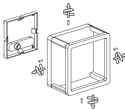
2. Untie screws & remove the lid
